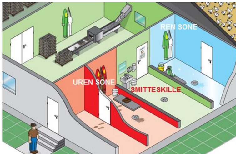
Prinsippkisse av tredelt smittesluse
